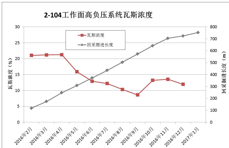
图 3-13: 2-104 工作面本煤层钻孔瓦斯浓度
